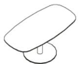
椭圆形茶几 DIP19.12 1000(W)*600(D)*400(H)
